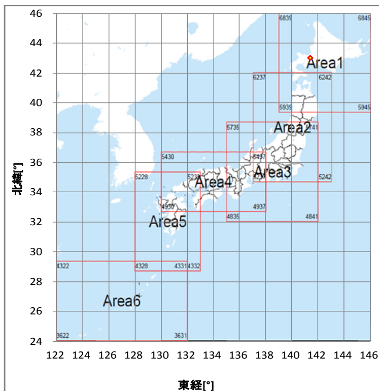
図 13 メッシュ農業気象データの 6 つのエリア
