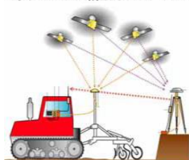
均平システム構成 (RTK-GPS)
