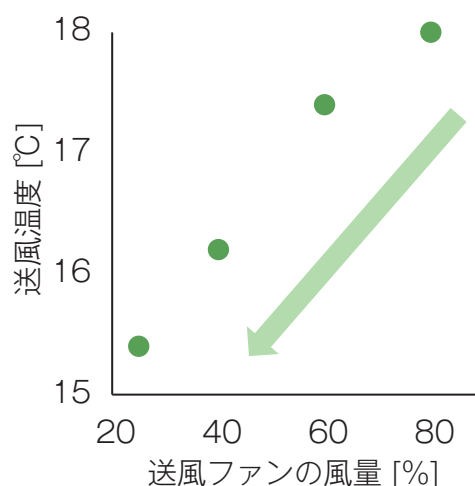
生葉コンテナ送風ファンの風量と送風温度との関係 ※外気温23.6℃の場合の例
