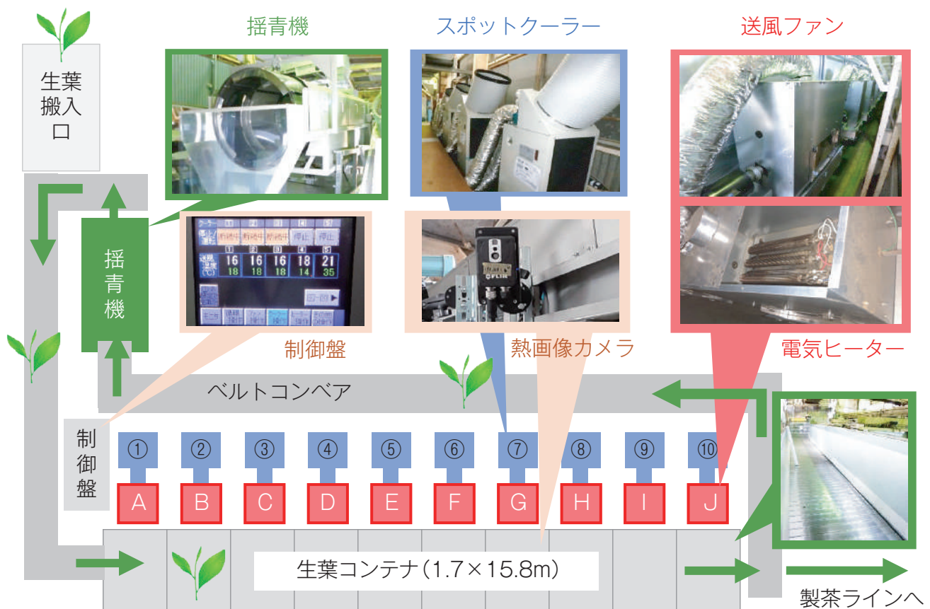
生葉低温保管を利用した「香り緑茶」生産設備の概要図
