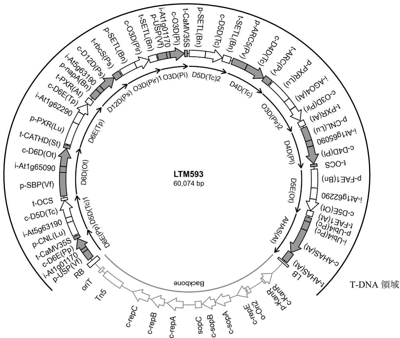
10 図 3 プラスミド LTM593 地図
