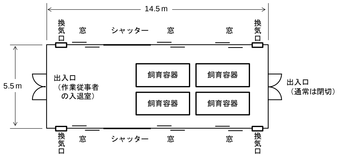
図 6. 隔離飼育区画内の飼育室の平面図
