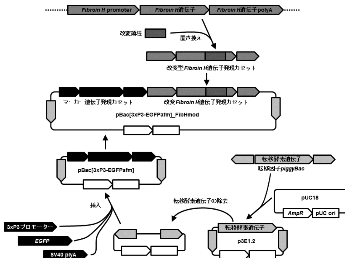
図 11. 改変 Fibroin H 遺伝子の導入に用いたプラスミド pBac[3xP3-EGFPafm]_FibHmod の作
