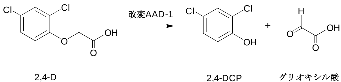
別添図3 改変AAD-1蛋白質の作用機作
