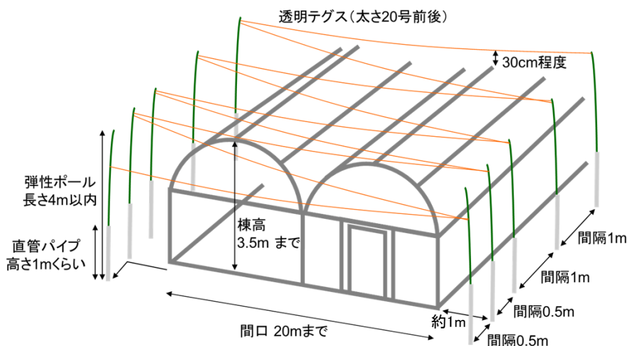
「ハウスにテグス君」の構造
