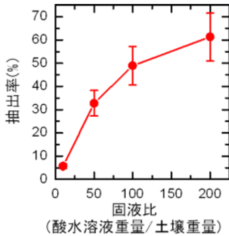
図 2 : 固液比によるセシウム抽出率の変化 土壤と 0.5 mol/L の希硝酸を混合し、 95 °C、45 分静置した際のセシウムイオン 抽出率
