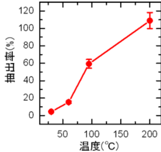
図 3 : 温度によるセシウム抽出率の変化 抽出温度を変化した際のセシウムイオン抽 出率 (0.5mol/L の硝酸、固液比 200) *抽出率が 100%を超えているのは、土壤中の セシウムイオン量のばらつきに起因する。
