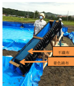
図4：除染フィルターによる実証試験
