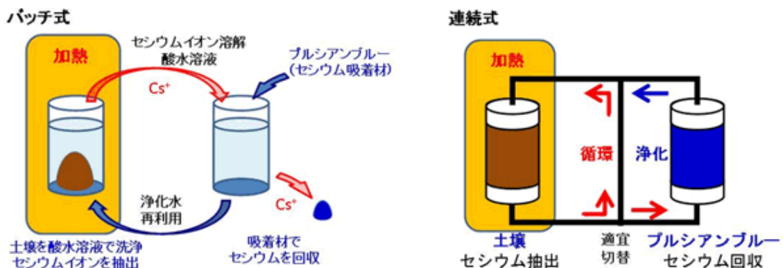
図1：土壌からの放射性セシウム抽出ー回収システムの模式図
