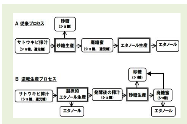
【砂糖・エタノール複合生産プロセス】
