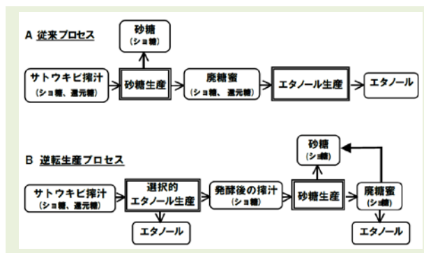
【砂糖・エタノール複合生産プロセス】
